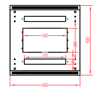
BOTTOM VIEW: 600*600
