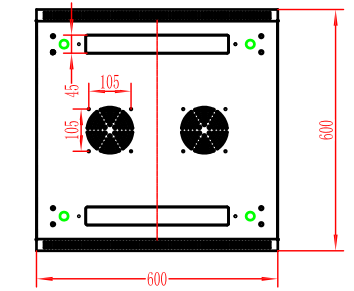
TOP VIEW: 600*600
