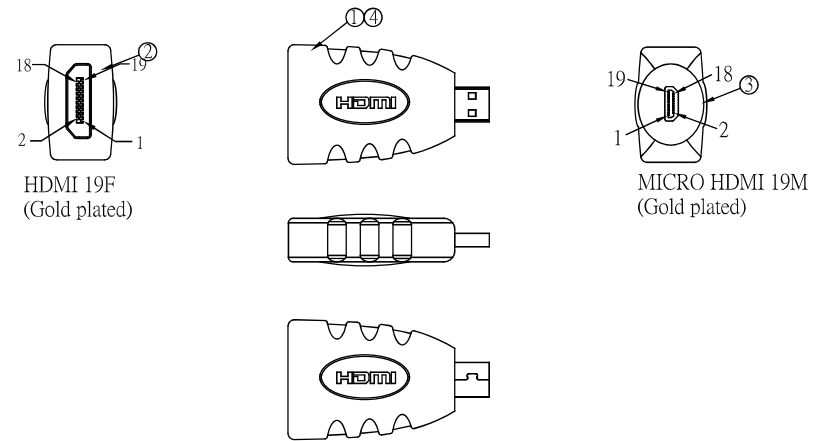
MICRO HDMI 19M TO MINI HDMI 19F ADAPTER Black Adaptor
